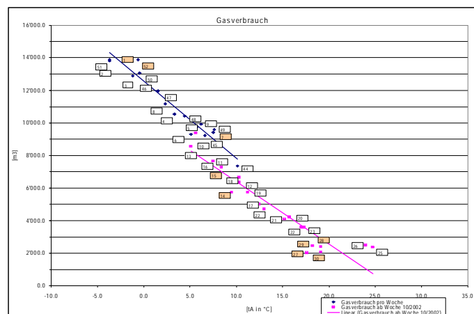
Gasverbrauch vor und nach ersten BO-Massnahmen
