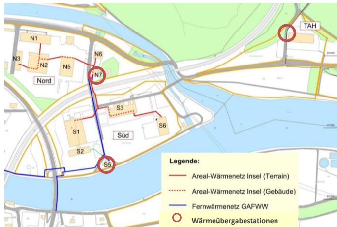
Situationsplan Wärmenetz Insel und Fernwärmenetz
